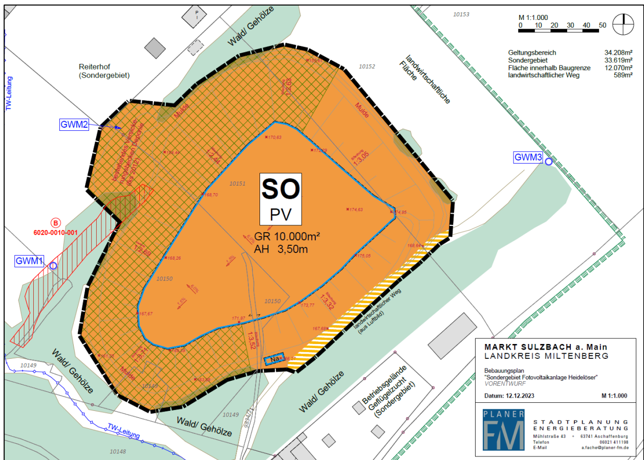
Abb. 2: Ausschnitt aus dem Bebauungsplan „Sondergebiet Fotovoltaikanlage Heidelöser“ (Planer FM, Stand: 12.12.2023)
