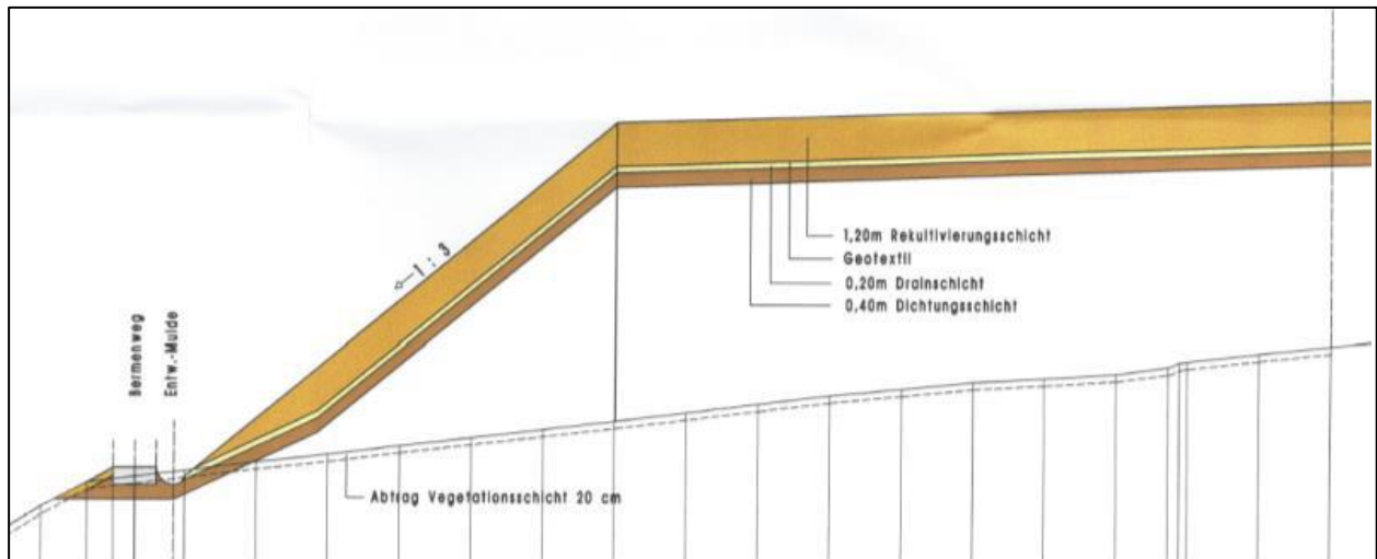
Abb. 6: Ausschnitt Längsprofil Deponieabdeckung (Planung fks 2001)
